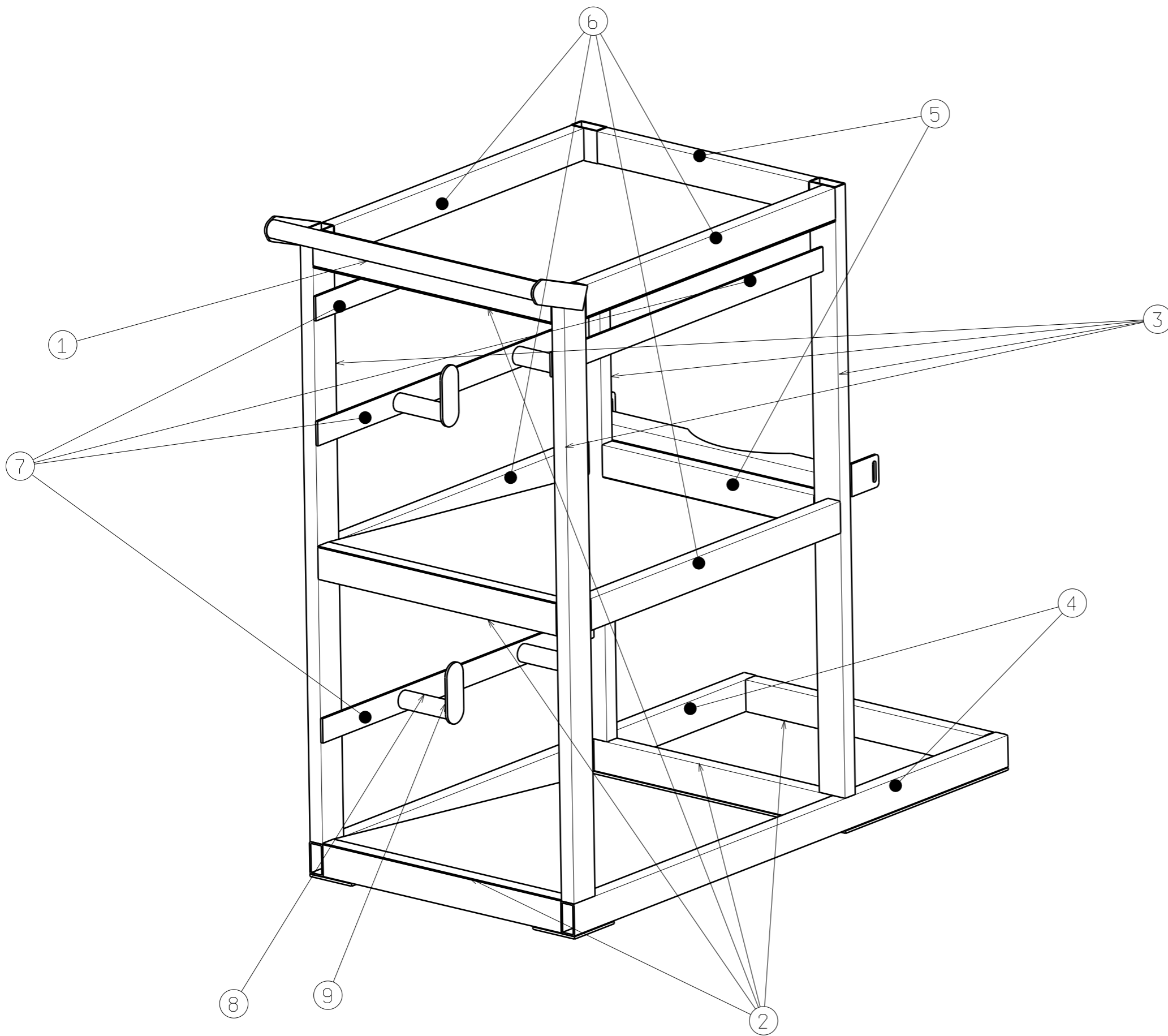
Isometric view Scale: 1:5
